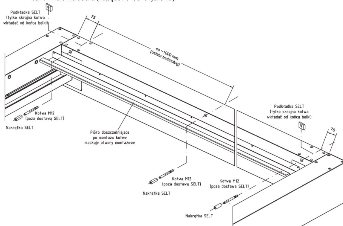
Rysunek 14 - Montaż przyścienny do belki tylnej/przedniej.
