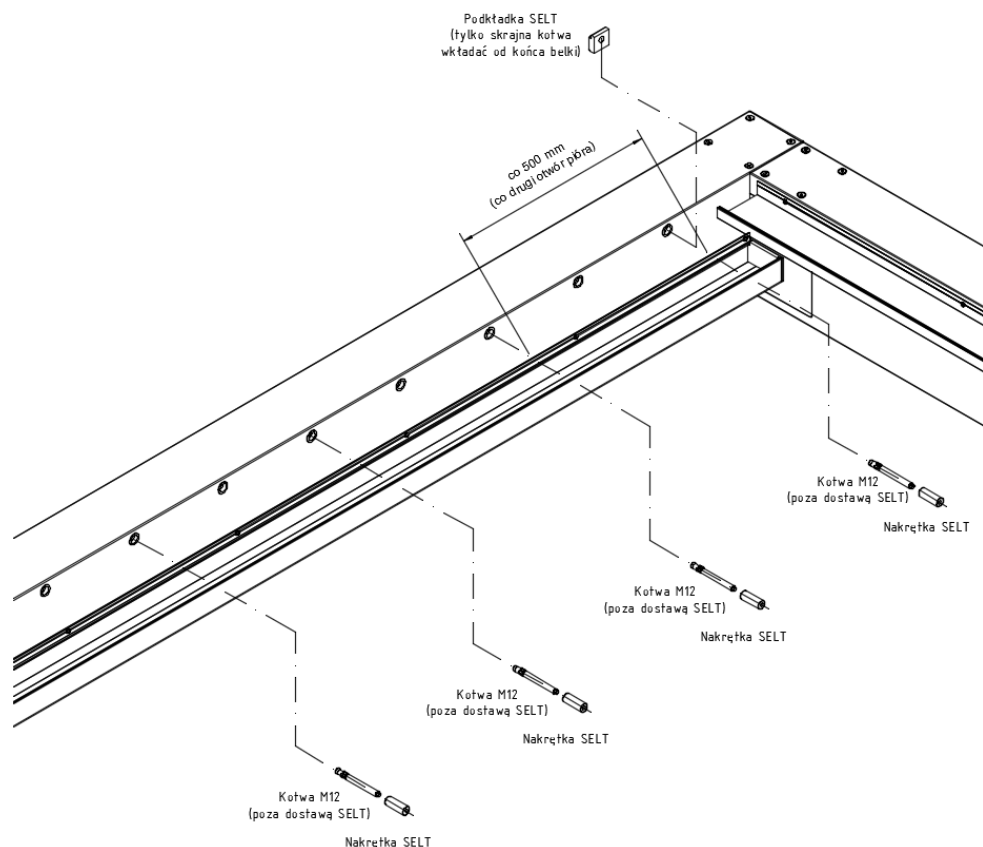
Rys. 4. Sposób zakotwień przyściennych na belkach wzdłużnych – rozwiązanie preferowane (alternatywnie możliwe na belkach poprzecznych). Odstępów mocowań w zakresie od 500 do 750 mm (na przedłużeniu otworów)-wg technologii
