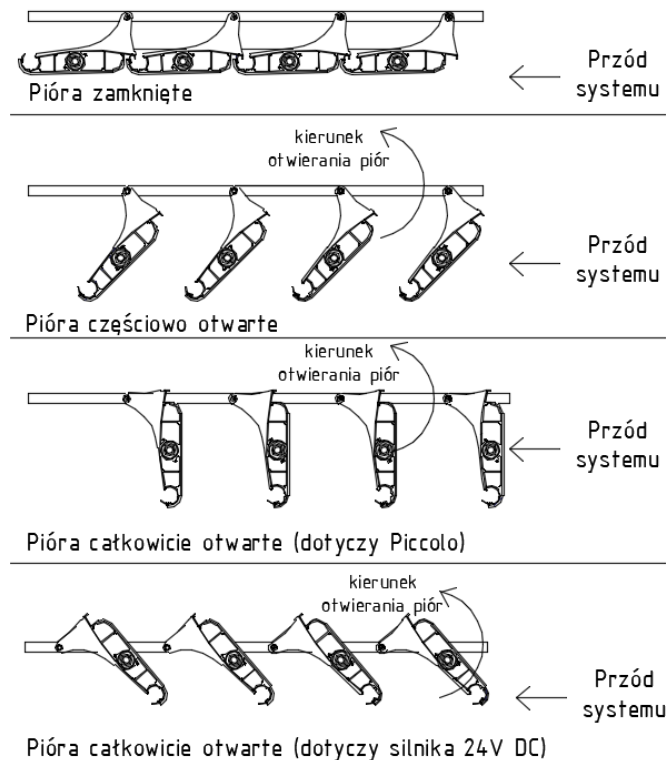
Rys. 3. Standardowe ustawienie kierunku otwierania piór w Pergoli SB500R.
