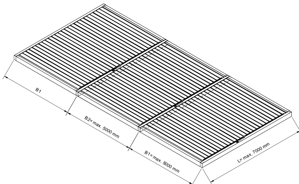
Rys. 2. Pergola SB500R modułowa - Wymiary gabarytowe: B1 – szerokość maksymalna modułu skrajnego, B2 – szerokość maksymalna (osiowa) modułu środkowego, L max – długość maksymalna, wysokość ramy wynosi 290 mm.
