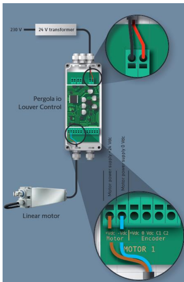
Rys. 33 Schemat obszarów podłączeń wewnątrz centralki Pergola io Louver (opisy na dolnym powiększeniu podano jako pogrubione w tabeli powyżej)
