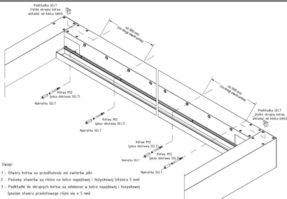
Rysunek 15- Montaż przyścienny do belki wzdłużnej. Odstępny mocowań w zakresie od 500 do 750 mm (na przedłużeniu otworów)-wg technologii
