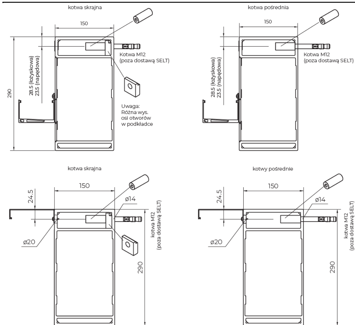
Rys. 6. Przekroje kotwien przyściennych SELT (u góry-belki wzdłużne, poniżej-poprzeczne)
