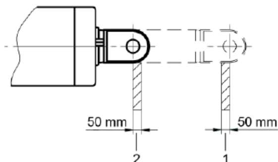
Rysunek 32 Dopuszczalna redukcja skoku silnika
